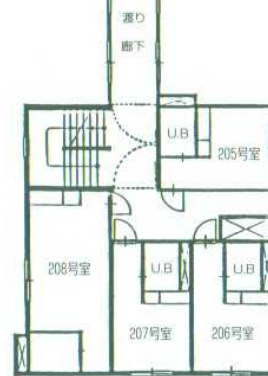
別館2階平面図
